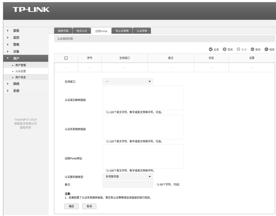
图4-12 远程Portal
